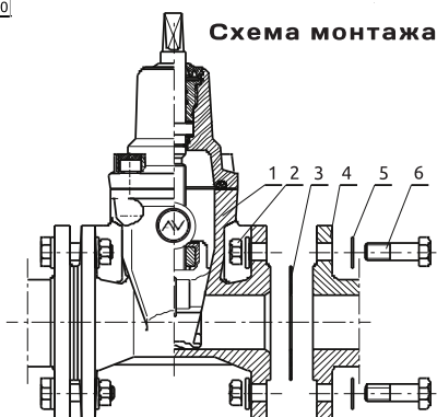
1. задвижка, 2. гайка, 3. уплотнитель, 4. фланец трубопровода, 5. шайба, 6. монтажный винт
